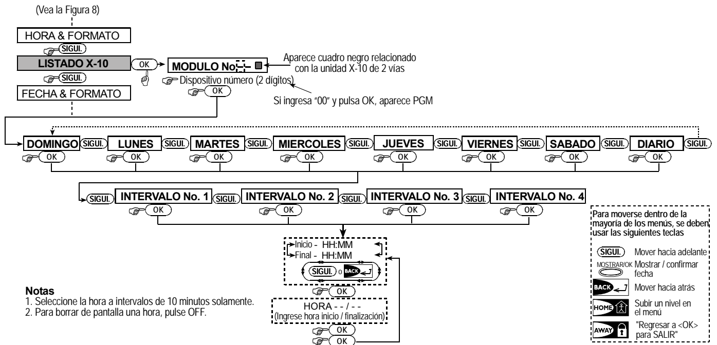
Figura 9 DETALLE "A" – Programación de dispositivos
